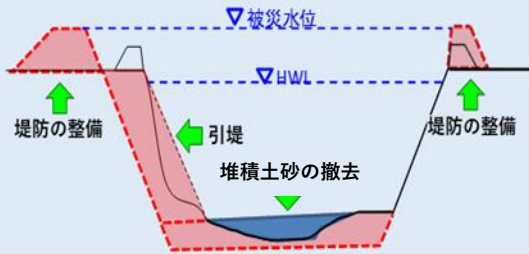
＜改良復旧イメージ断面図＞
