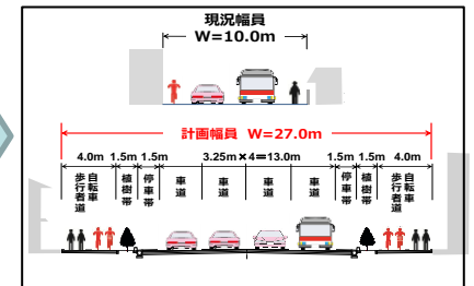
県道熊本高森線の4車線化計画
