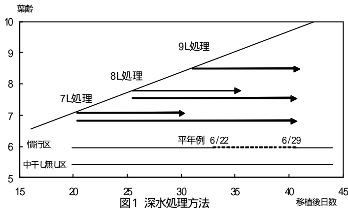
図1 深水処理方法
