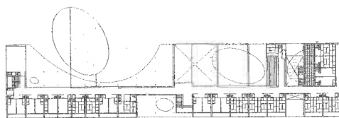
2階平面図
