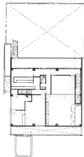
2階 平面図
