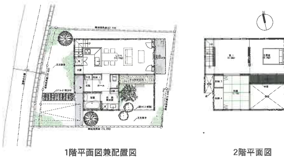
1階平面図兼配置図
