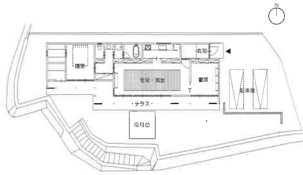
平面図
