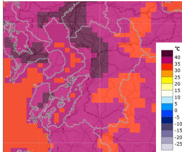
3日日中の最高気温（予想）
