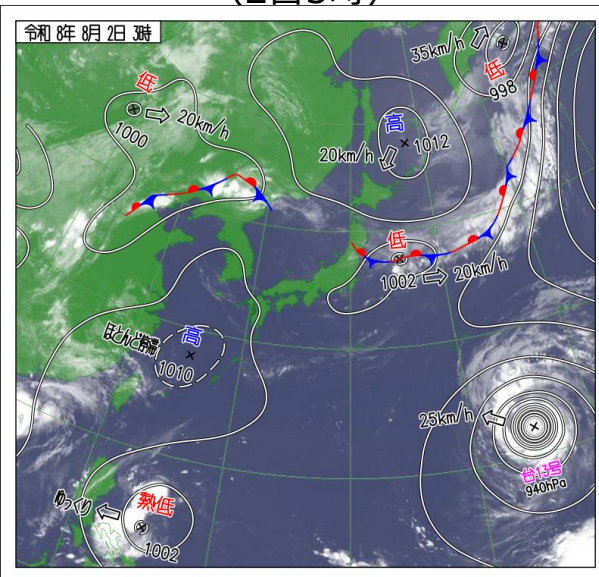
衛星赤外画像と地上天気図 (2日3時)
