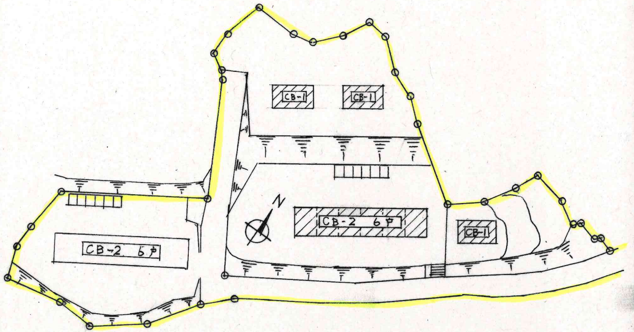
本渡第二教職員住宅 敷地現況図
