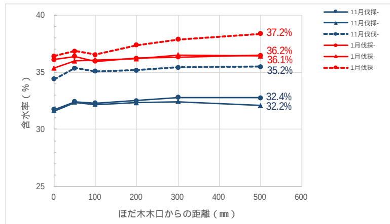
図 - 1 原木の長さ方向の含水率分布
