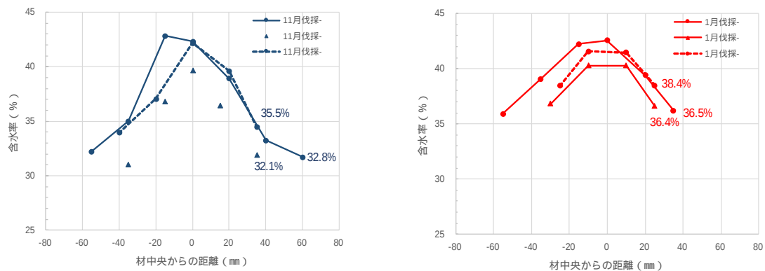
図 - 2 木口から500mm位置の横断面方向含水率 (湿量基準) 分布
