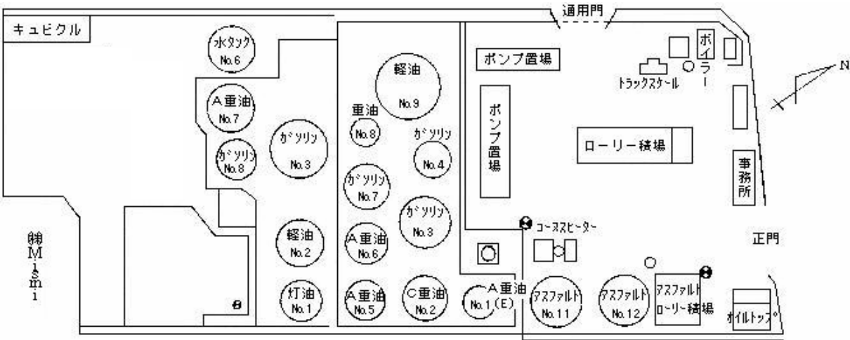
図1 東西オイルターミナル八代油槽所 A地区本庫配置図
