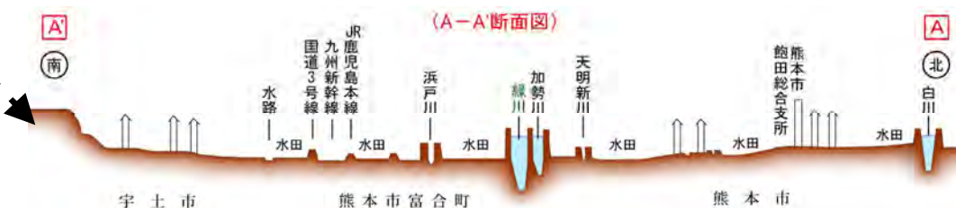
図 1.1-4 緑川堤内地横断図
