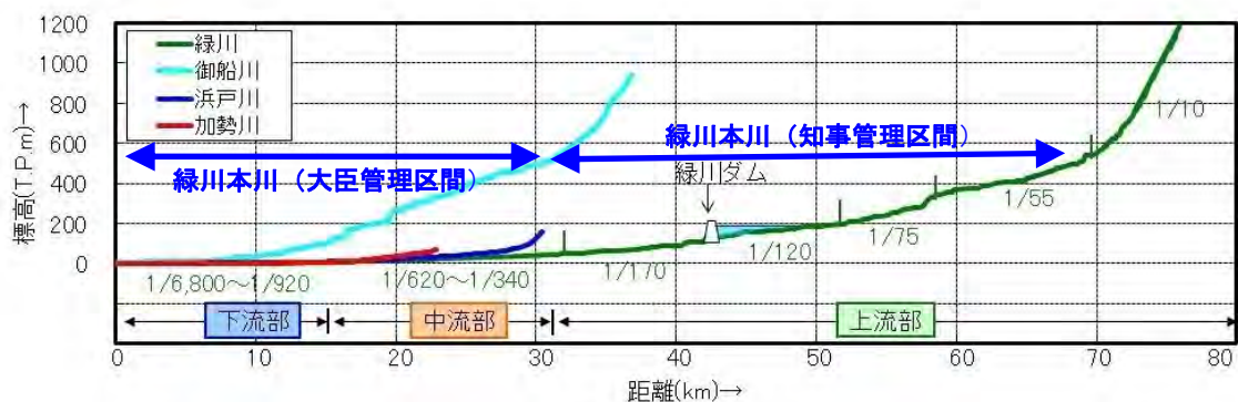
図 1.1-3 河床勾配縦断図
