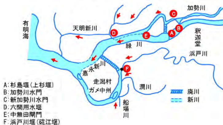
図 1.2-2 緑川第一期改修概要図
