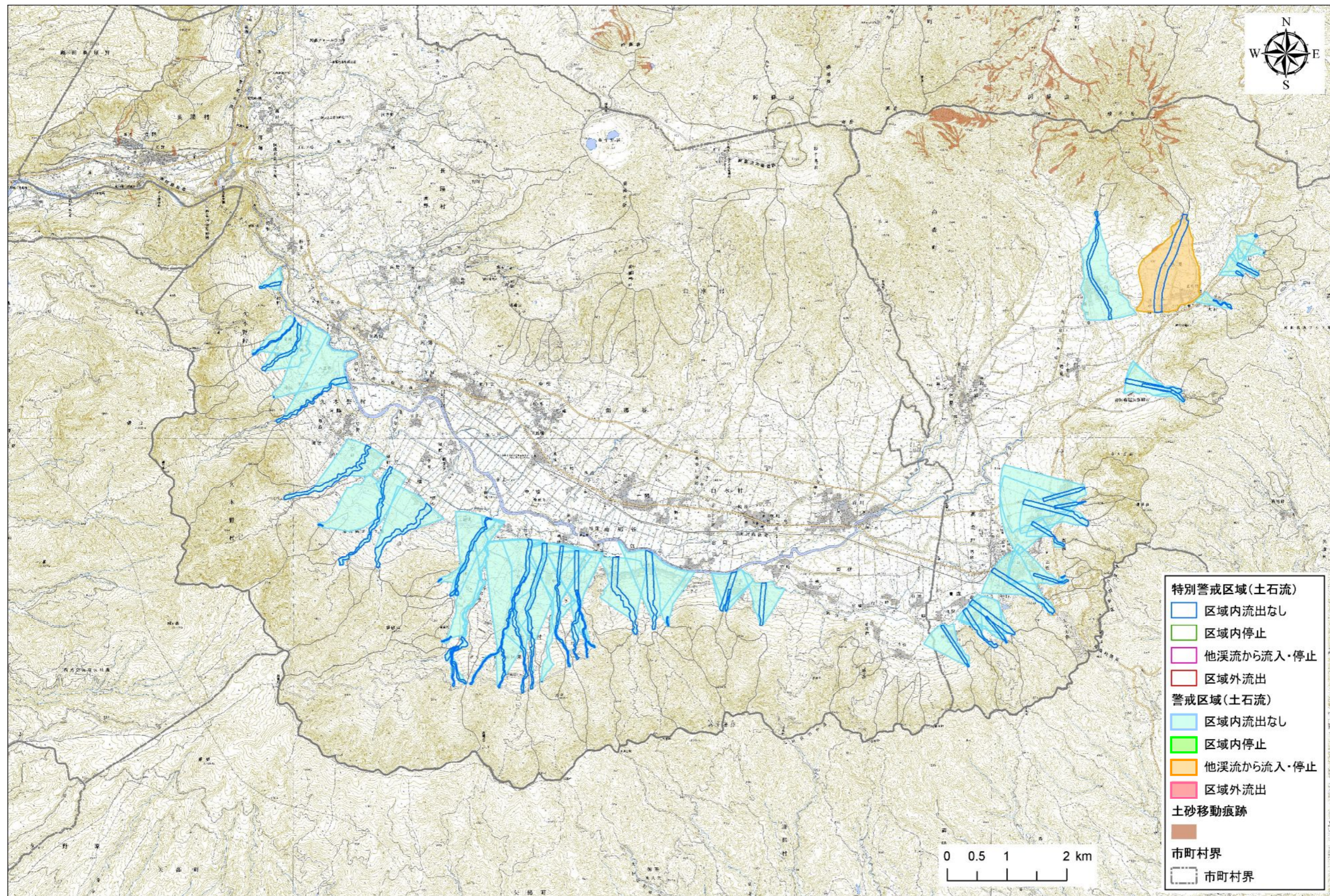
図 3.4 土砂災害警戒区域、土砂災害特別警戒区域及び土砂移動痕跡の分布(阿蘇山南部)
