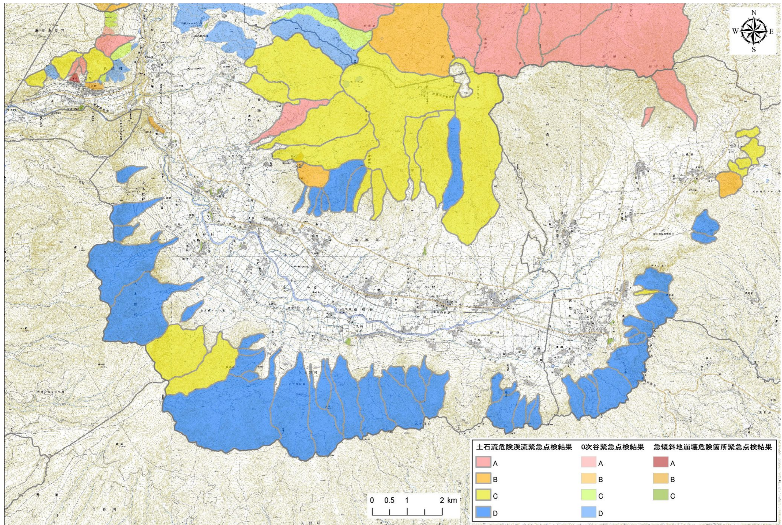
図 2.4 緊急調査結果位置図 阿蘇山南部
