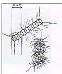
キートセロス属 Chaetoceros spp.
