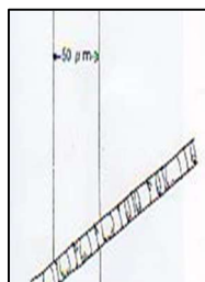
スケルトネマ属 Skeletonema spp.
