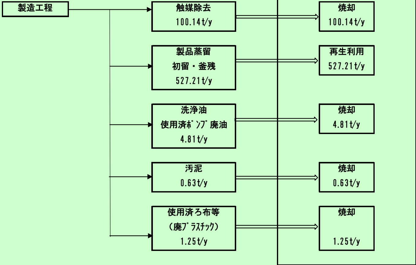
一般産業廃棄物処理フローシート (R.4年度実績)
