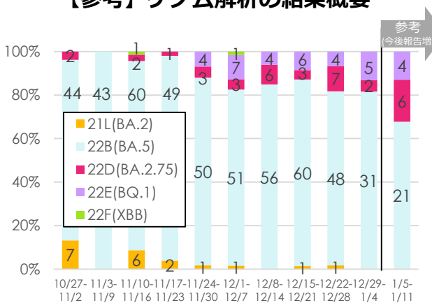
PANGO系統について、Nextstrain clade別に集計。 結果判明までのタイムラグがあるため、日付が近い値は変動する。
