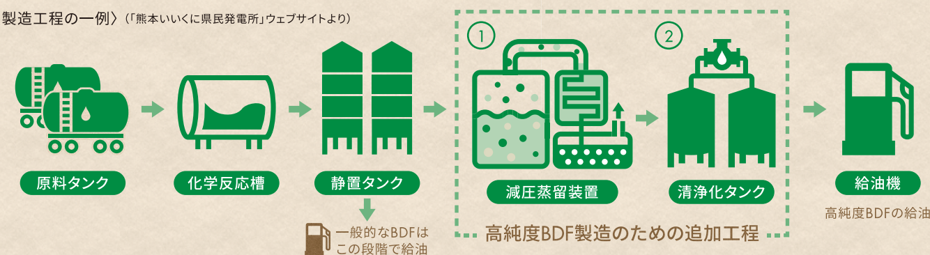
〈製造工程の一例〉(「熊本いづくに県民発電所」ウェブサイトより)
