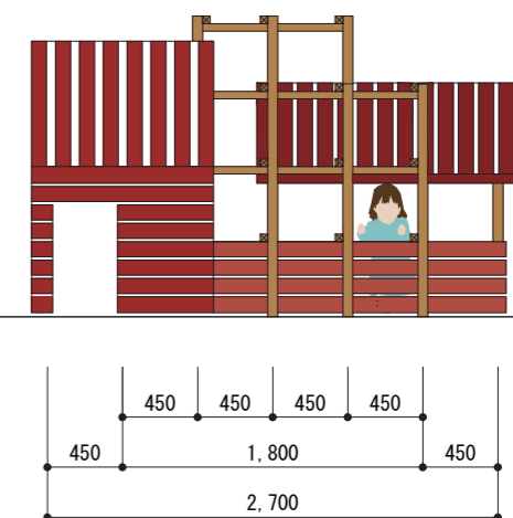
東立面図
