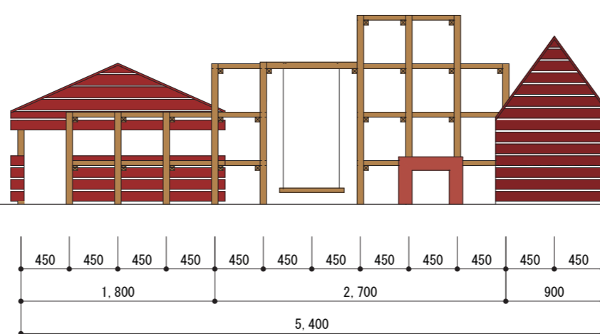
南立面図
