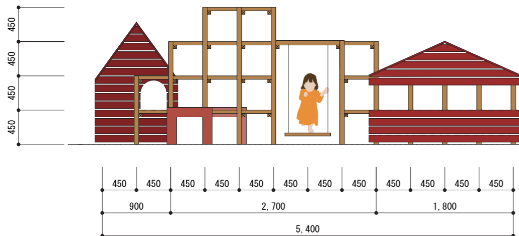
北立面図
