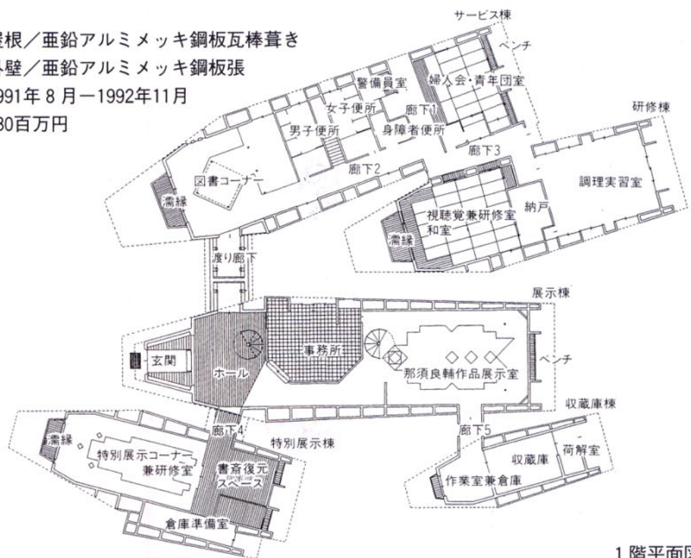
1階平面図
