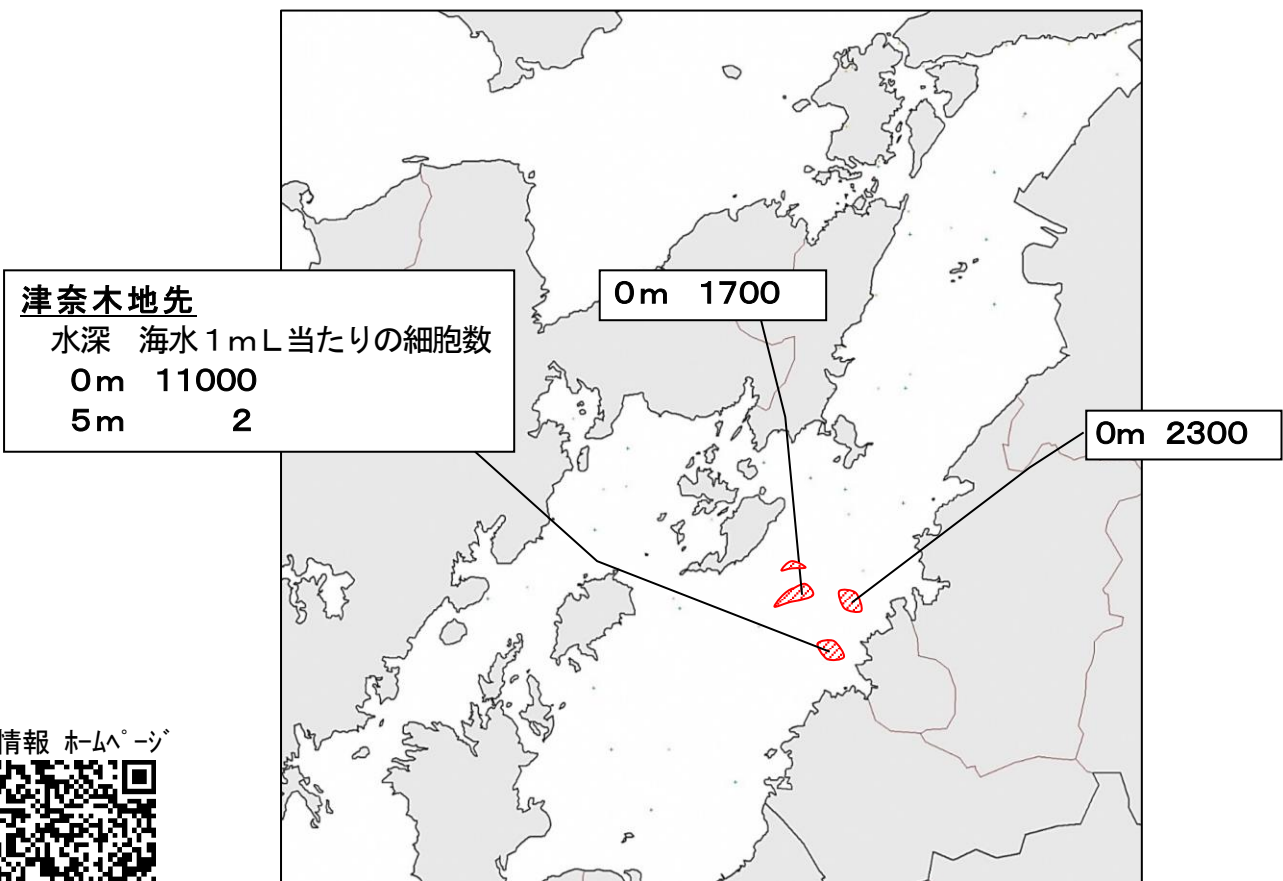
図 赤潮発生海域
