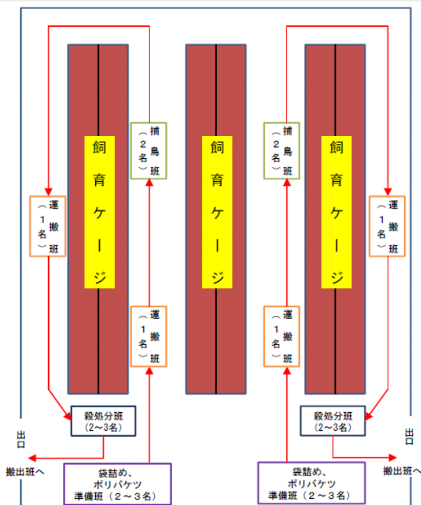
ケージ式家きん舎内の作業動線の例
