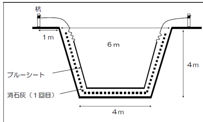
埋却溝の例（ブルーシートを敷設した場合 出典：宮崎県）
