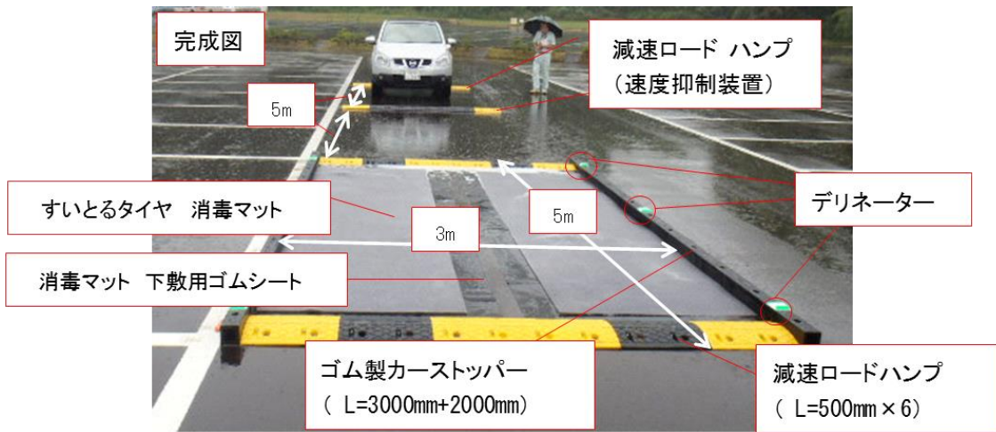
組立型車両消毒槽
