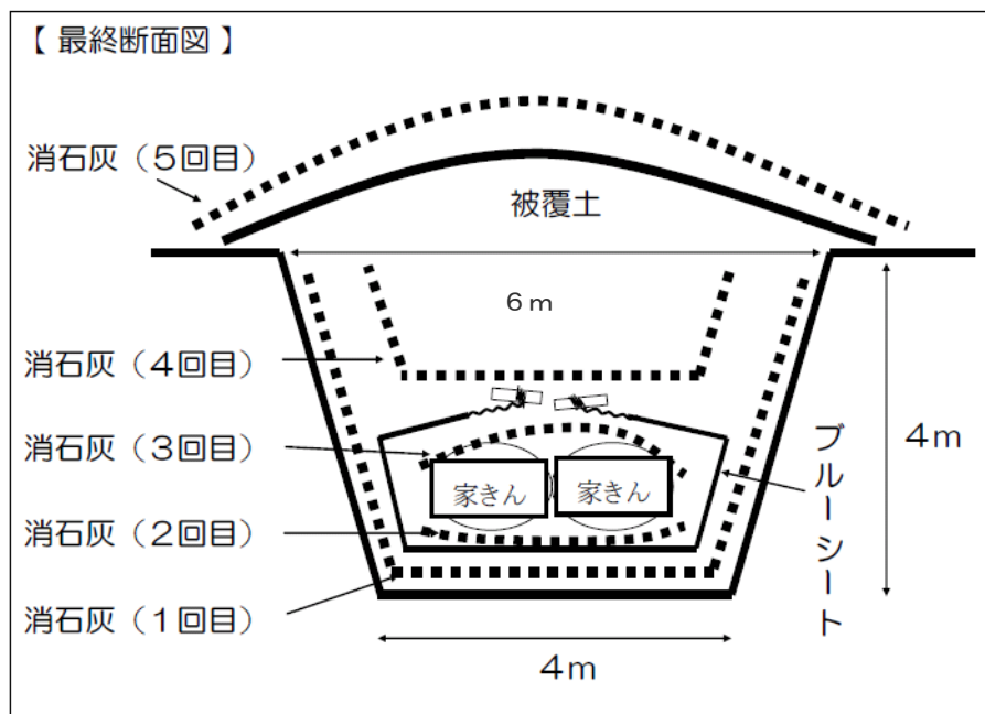
覆土後の埋却溝の例（ブルーシートを敷設した場合）
