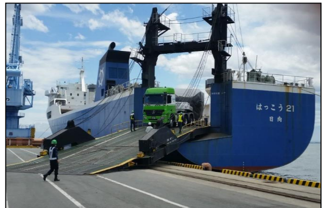
RORO 貨物荷役状況
