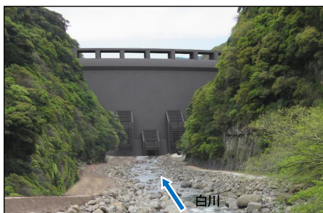
上流側からダムを望む
