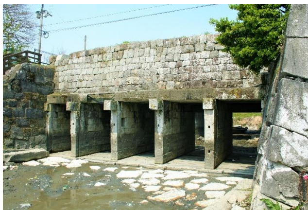
6. 大鞘樋門群(殻樋)
