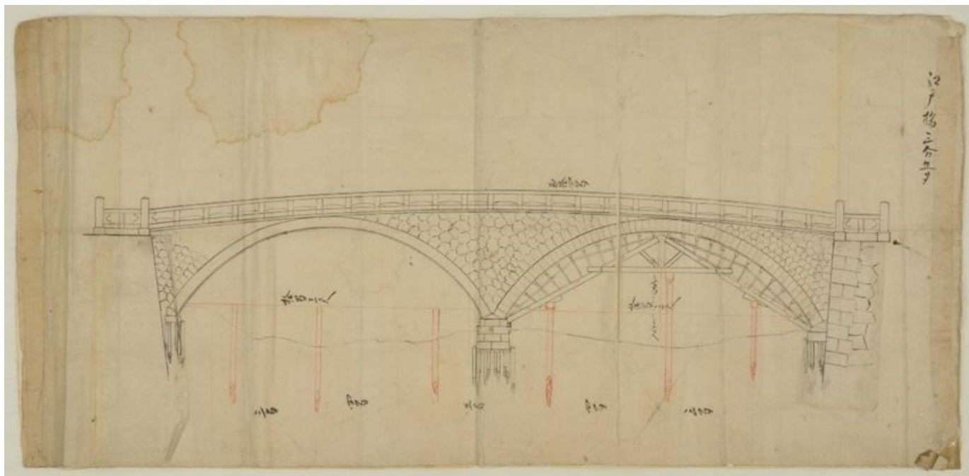
19. 橋本家文書(東京・江戸橋の設計図。江戸橋は勘五郎が熊本に戻った後の明治8年(1875)5月に完成。)
