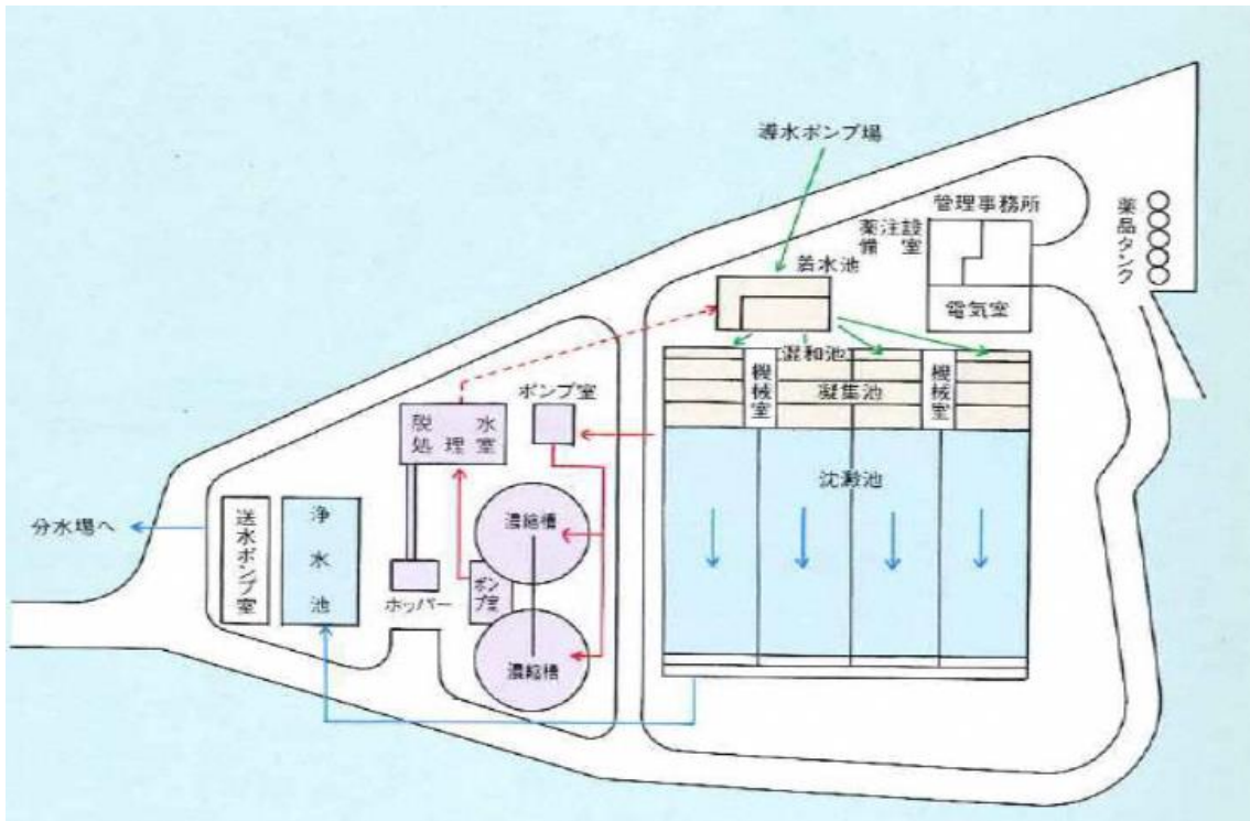
図表 10 施設配置図 (上の原浄水場)
