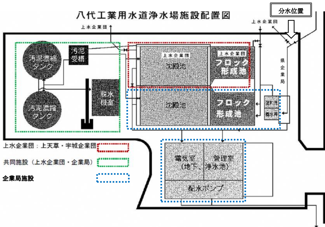
図表 13 施設配置図（白島浄水場）
