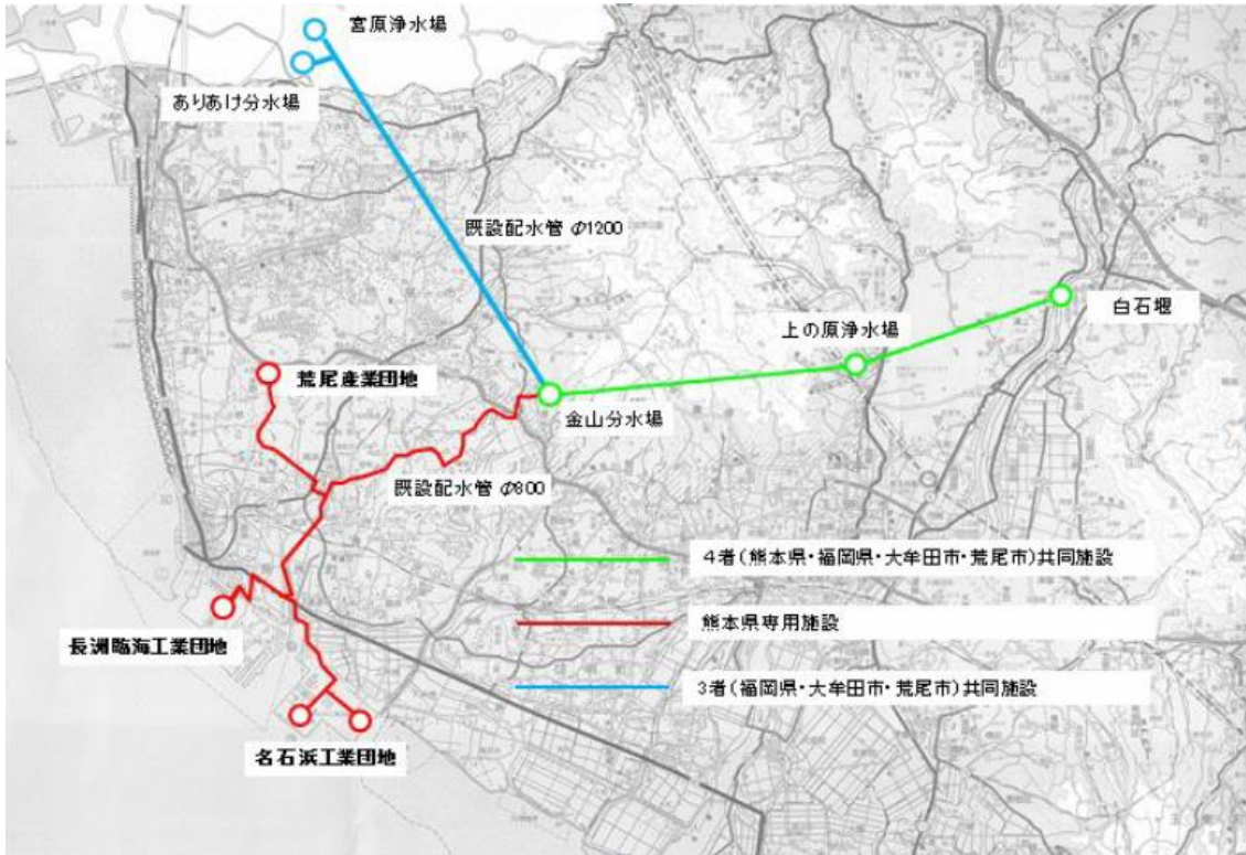
図表 9 配管図 (有明工業用水道)
