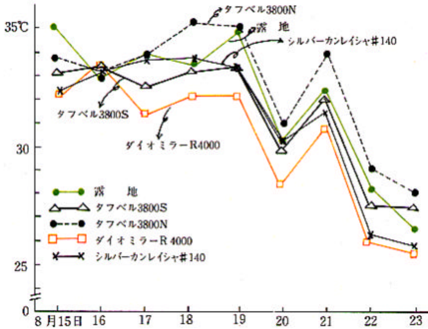
図1 トンネル内の最高気温
