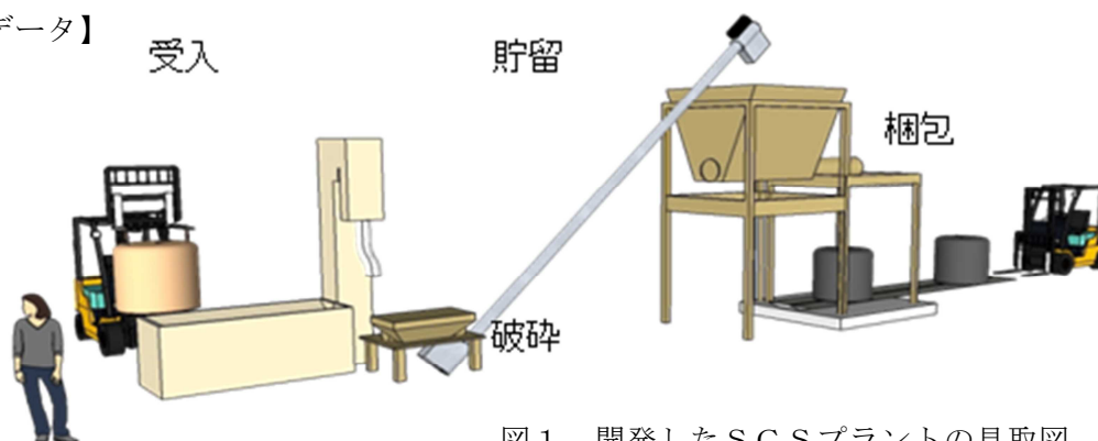
図1 開発したSGSプラントの見取図
